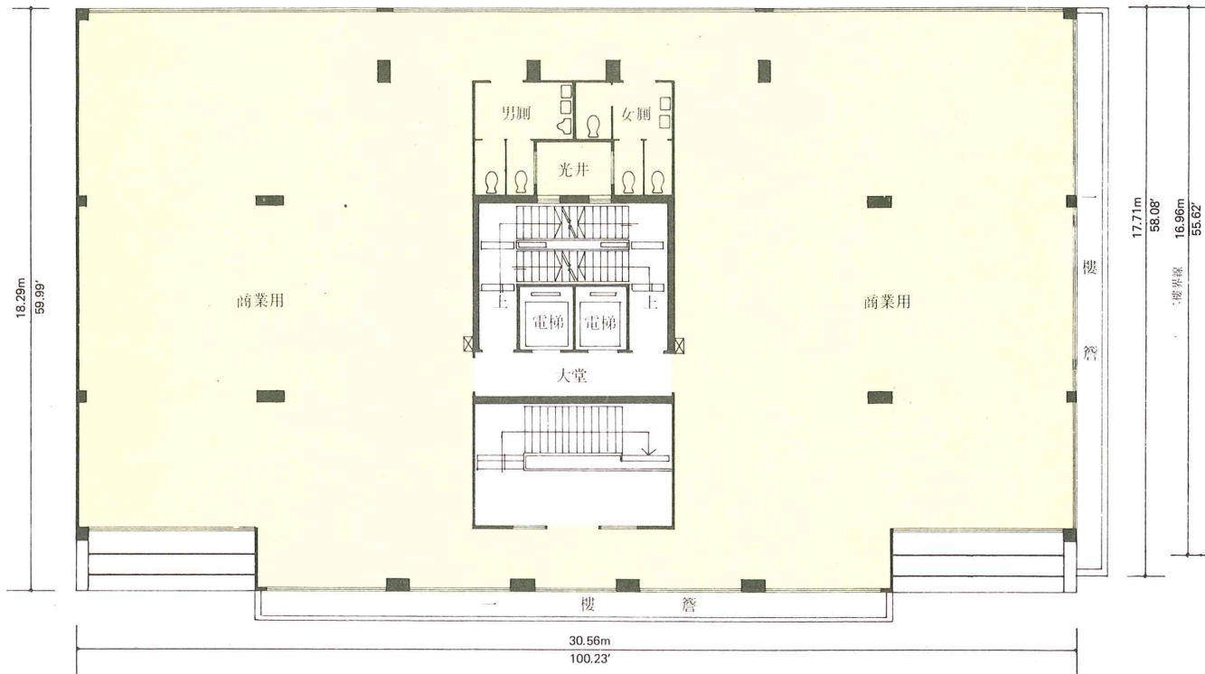
一樓至二樓平面圖
